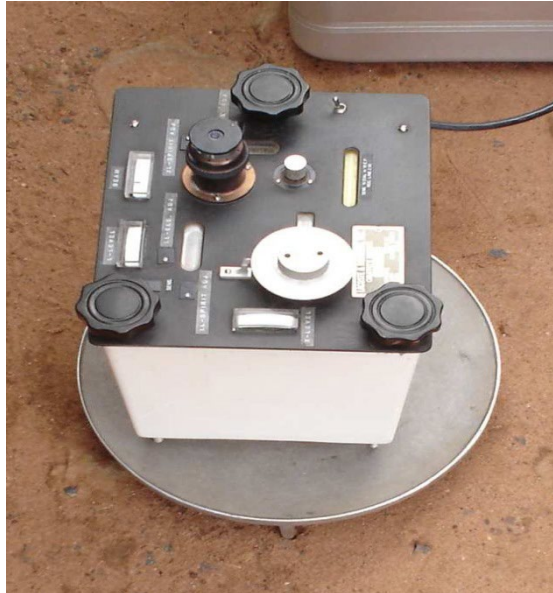
Gravímetro Lacoste & Romberg, modelo G, serie N° 1004
